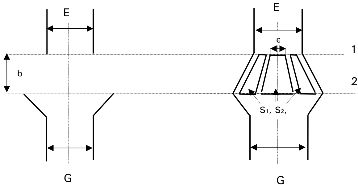
Figuur 1: Uitvoering aansluiting afvoer
